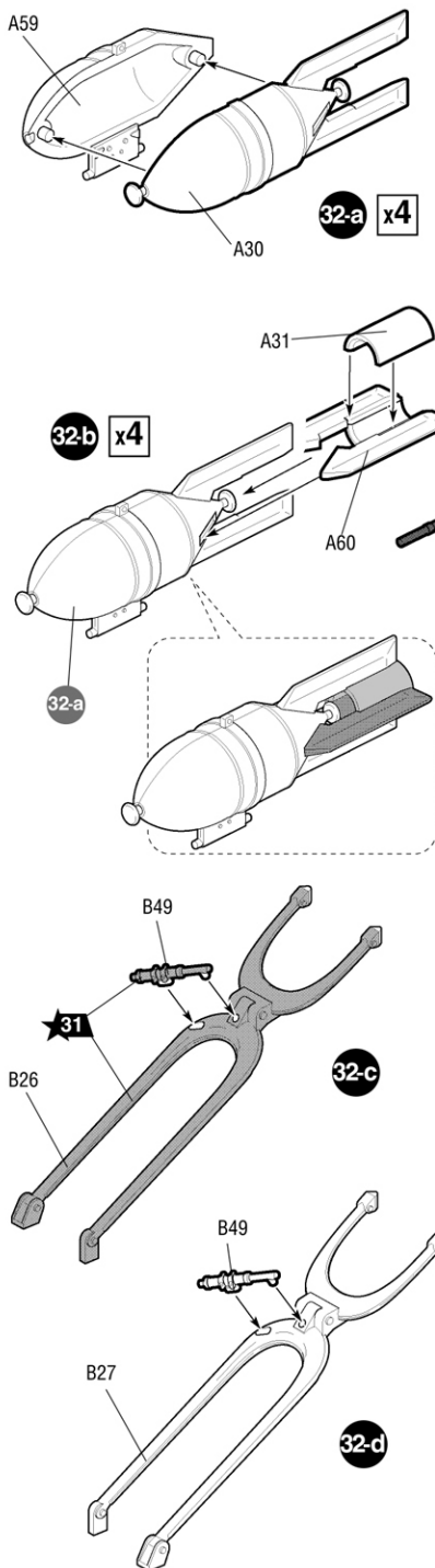
2 ВАРИАНТ СБОРКИ ASSEMBLING VERSION 2
