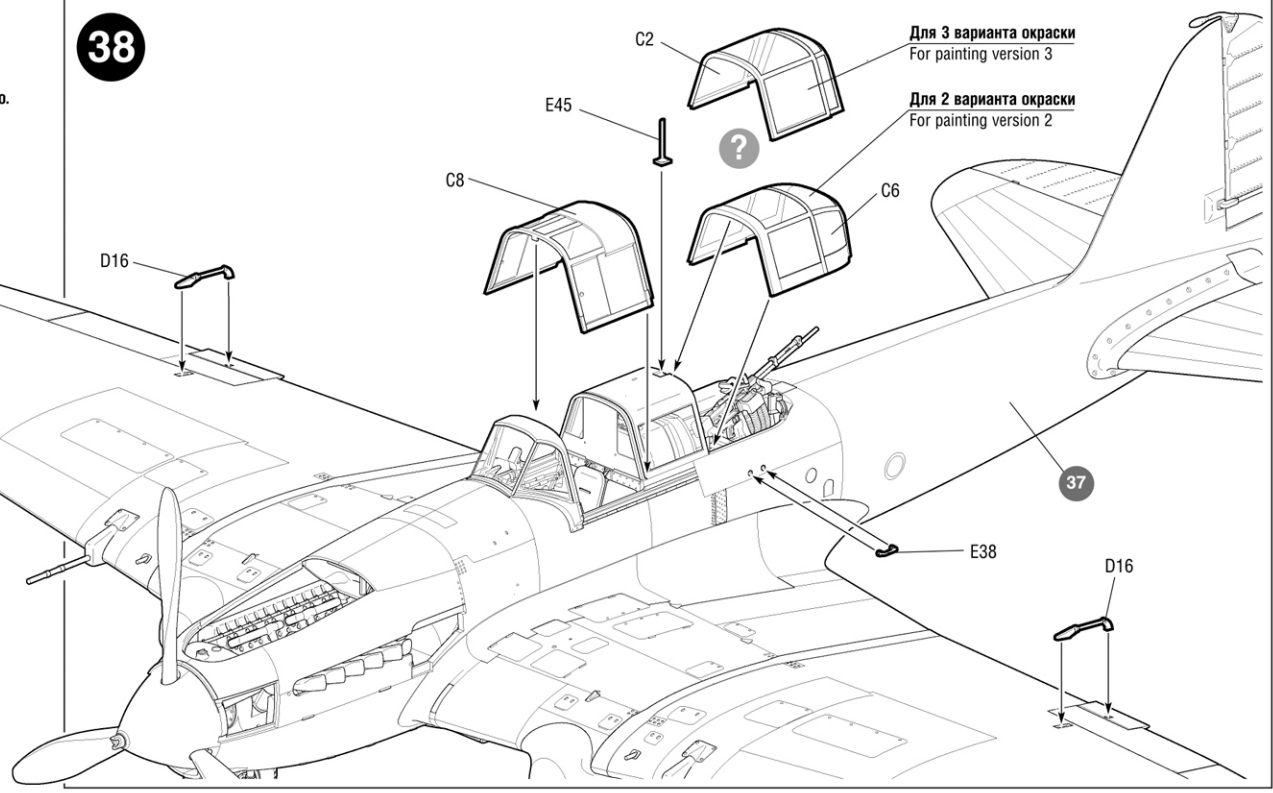
2 ВАРИАНТ СБОРКИ ASSEMBLING VERSION 2
