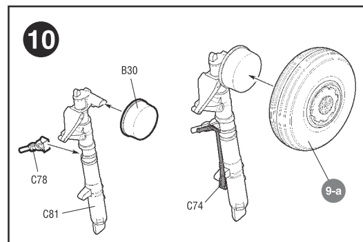
ВАРИАНТЫ СБОРКИ 1, 3 ASSEMBLING VERSIONS 1, 3
