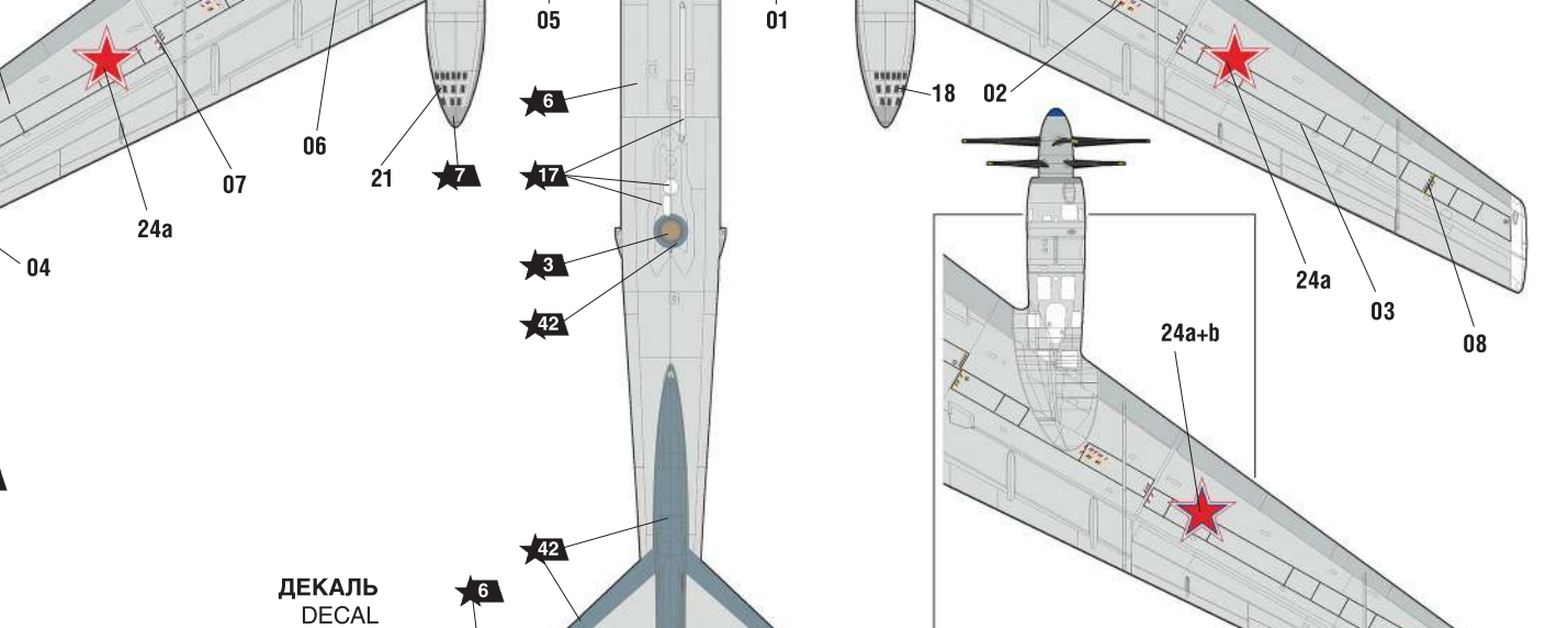
Ту-95МС «Самара» из состава Дальней Авиации ВВС России, 2014 г. Tu-95MS "Samara" of the Russian Air Force's Long Range Aviation, 2014.
