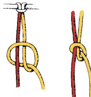
Рис. 23. Армянский узел
