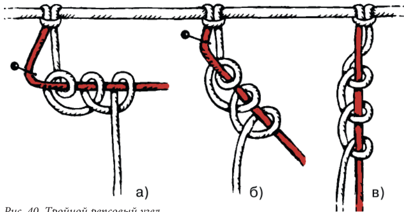
Рис. 40. Тройной репсовый узел
